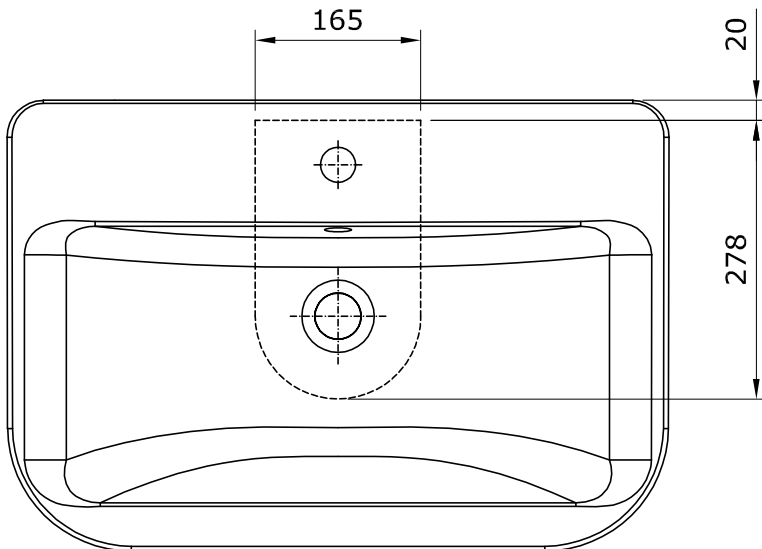
136370 - lavat.Look 66
