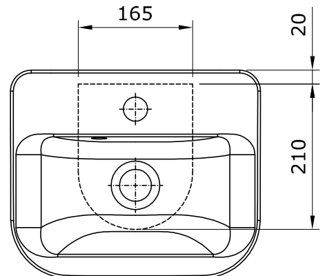
136300 - lava-mão Look
